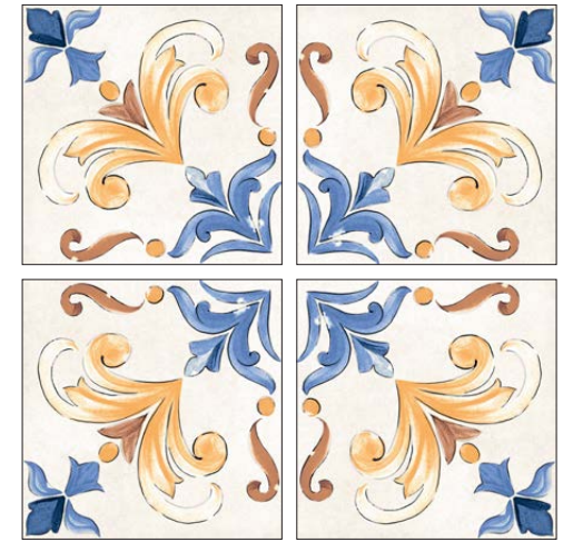
DECO A
