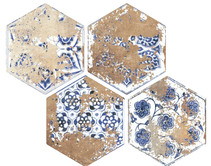
DECO MIX
