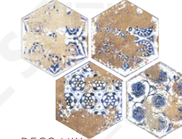
DECO MIX
